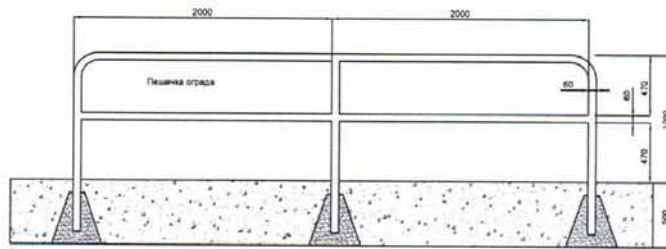
Скица пешачке ограде (Позиција 8.3.) са основним димензијама датим у милиметрима
